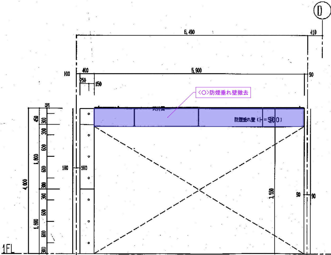
AGV走行路 d面
