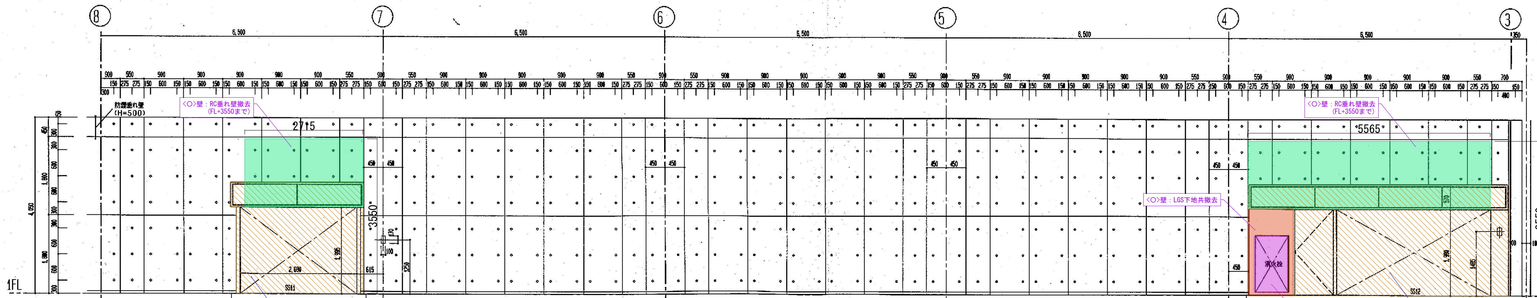
AGV走行路 a面
